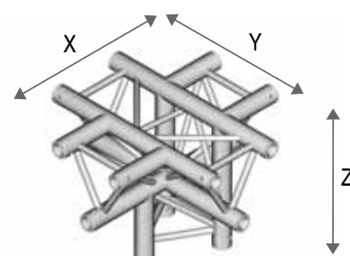
INCROCIO 90° CINQUE VIE VERTICE BASSO
