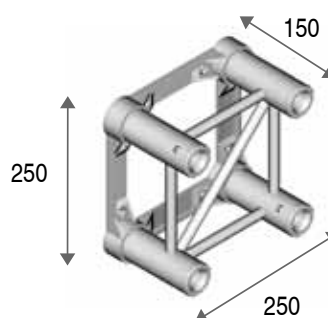
ADATTATORE QUADRO SUPERLITE PER STANDARD-ELITE 25
