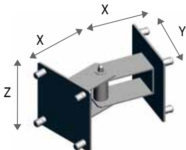
ANGOLO DUE VIE VARIABILE QUADRO
